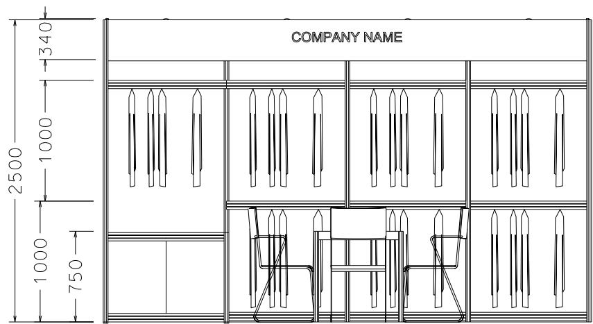
ELEVATION
